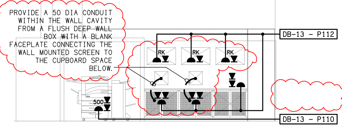
DETAIL C AV WALL ELEVATION 2 SCALE 1:50
