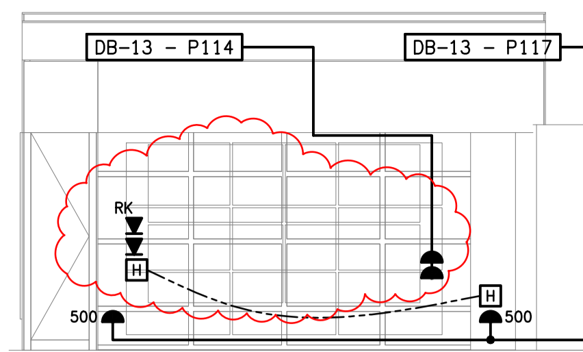
DETAIL B AV WALL ELEVATION 1 SCALE 1:50
